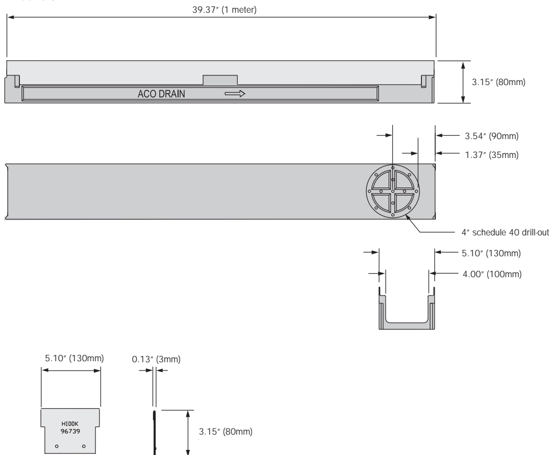
H100KS-8
